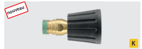
TR22 M : M22 F. Variante pour adaptateur 2+3. Laiton. Rotatif. Max. 400 bar / 150° C
