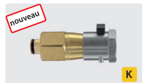
TR22 F : Coupleur femelle Ø 11 mm. Laiton/inox Max. 400 bar / 150° C
