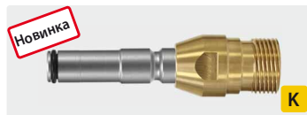
ST-247 : TR22 AG. Латунь/Нерж. сталь. Макс. 400 bar / 150° C
