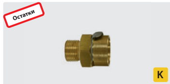
Муфта-штекер 10 мм : 3/8" AG. Макс. 400 bar
